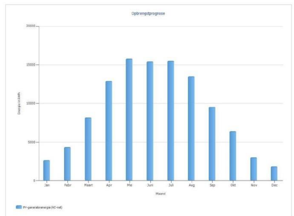
Afbeelding: Opbrengstprognose
